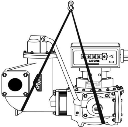
Şekil 11. Sayacın Taşınması
