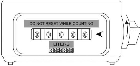
Şekil 7. Mekanik Numaratör
