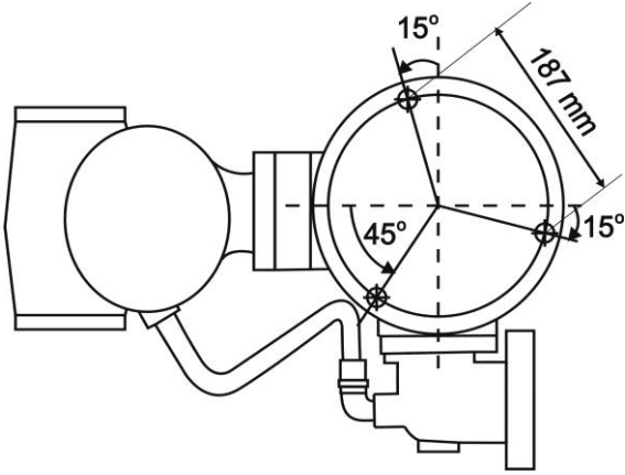
Şekil 3. Sayaç Alttan Görünüşü
